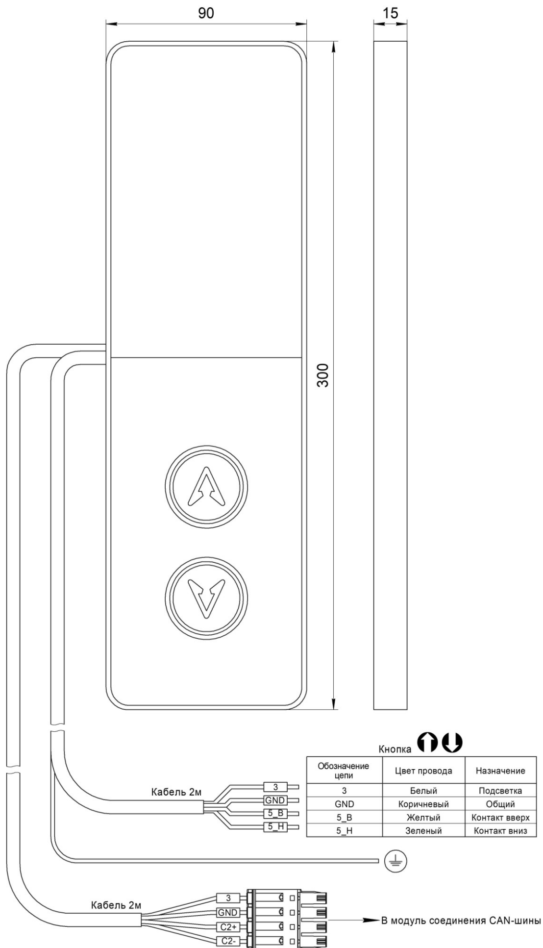
Рис.1 Внешний вид Вызывной пост ОПАЛ НШЕК.468381.057
